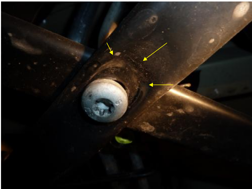
Diagonalstreben am Unterboden verschoben
